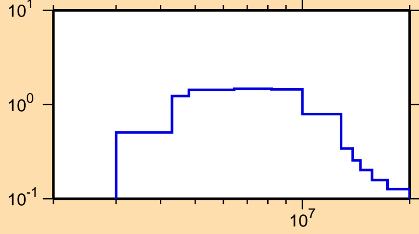
\sigma vs. E for ^{76}\text{Ge}(n,n\text{cont.})
