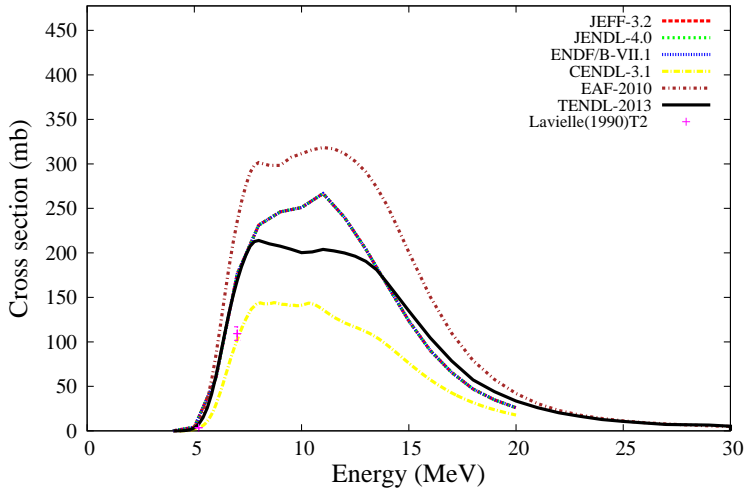
^{26}\text{Mg}(n,a)^{23}\text{Ne}
