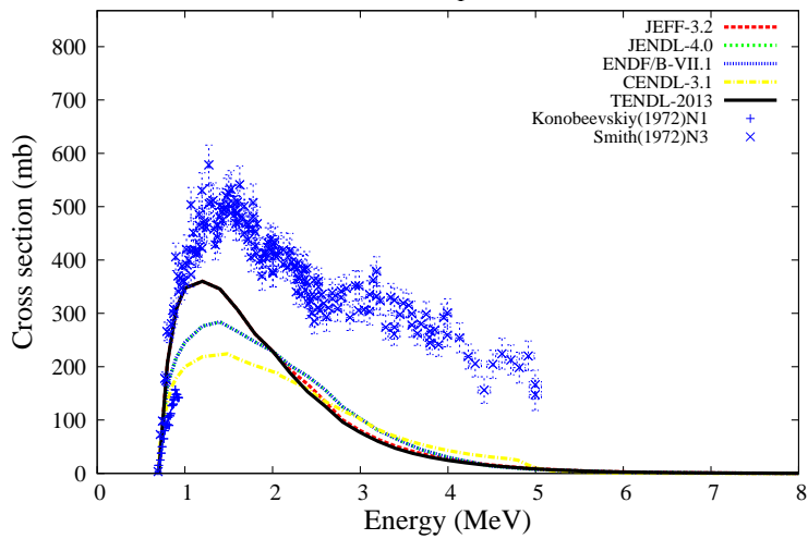
^{72}\text{Ge}(n,n_1')^{72}\text{Ge}
