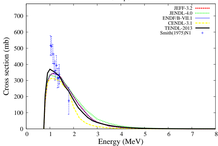
^{98}\text{Mo}(n,n_1)^{98}\text{Mo}
