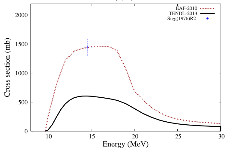
^{128}\text{Xe}(n,2n)^{127g}\text{Xe}
