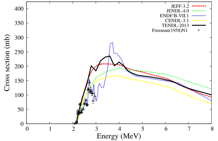
^{28}\text{Si}(n,n_2')^{28}\text{Si}
