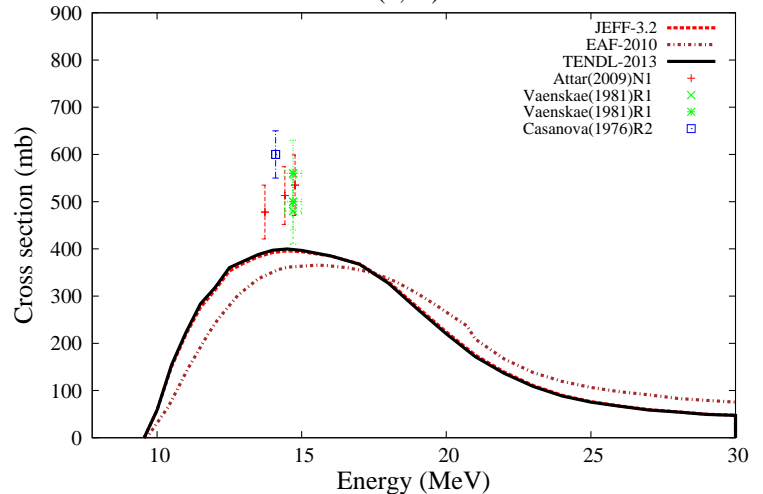
^{76}\text{Ge}(n,2n)^{75g}\text{Ge}
