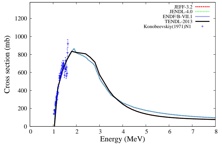
^{70}\text{Ge}(n,n_1')^{70}\text{Ge}
