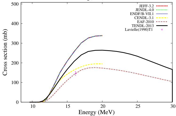
^{24}\text{Mg}(n,\alpha)^{20}\text{Ne}
