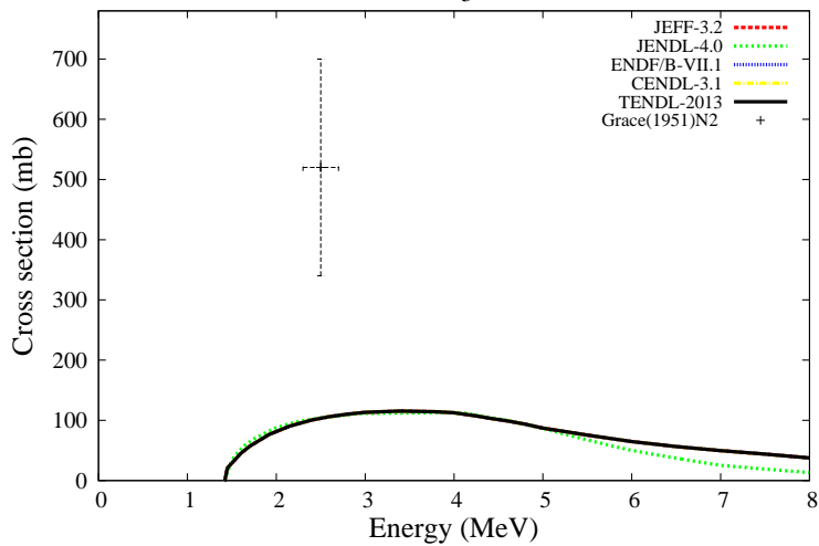
^{27}\text{Al}(n,n_3')^{27}\text{Al}
