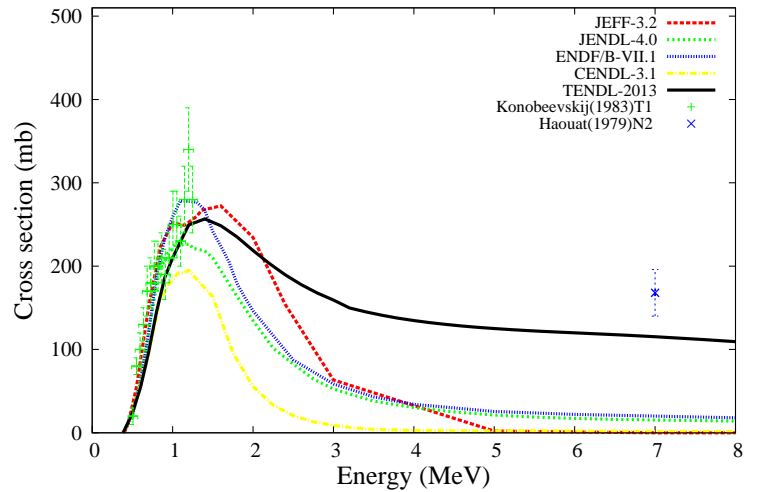
^{154}\text{Sm}(n,n_2')^{154}\text{Sm}
