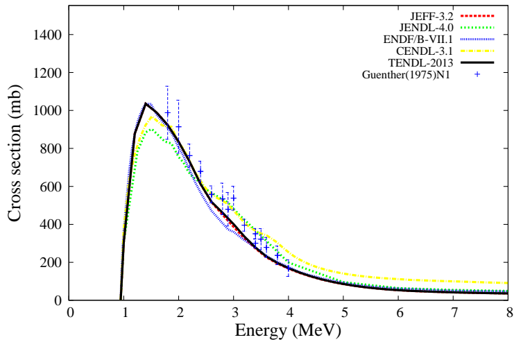
^{94}\text{Mo}(n,n_1)^{94}\text{Mo}
