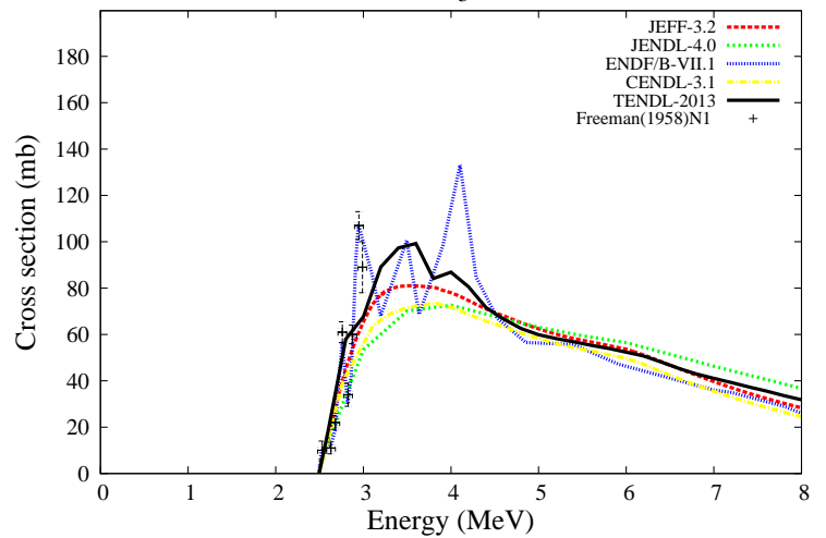
^{28}\text{Si}(n,n_3')^{28}\text{Si}
