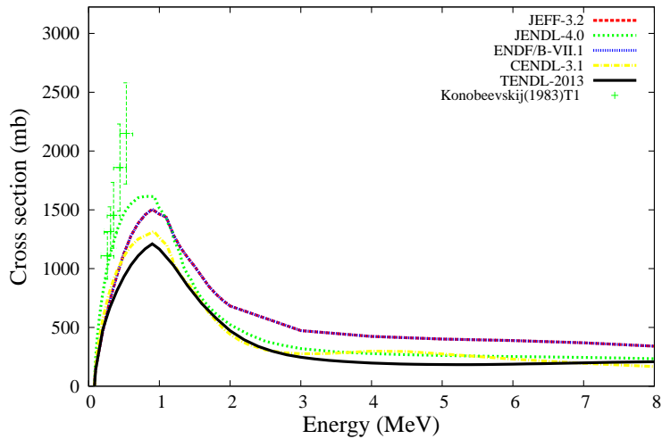
^{156}\text{Gd}(n,n_1)^{156}\text{Gd}
