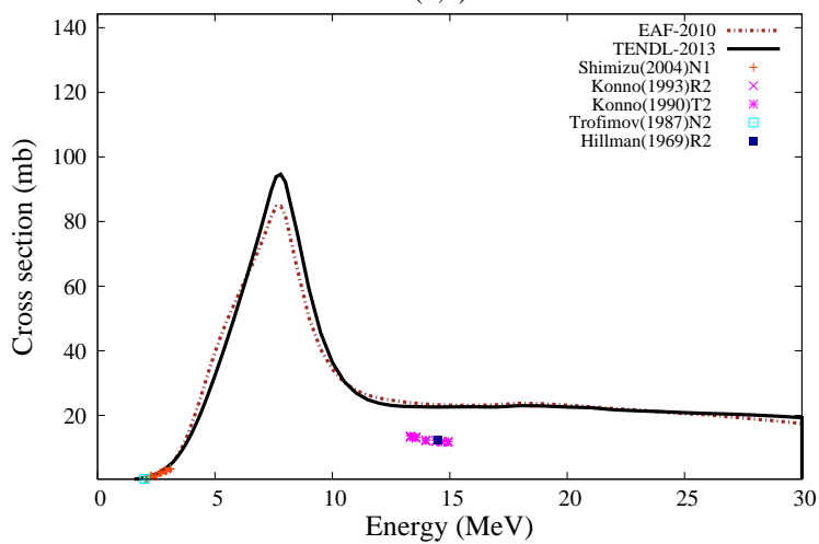
^{\text{nat}}\text{W}(n,n)\text{W}
