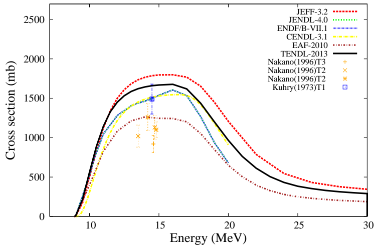
^{126}\text{Xe}(n,2n)^{125}\text{Xe}
