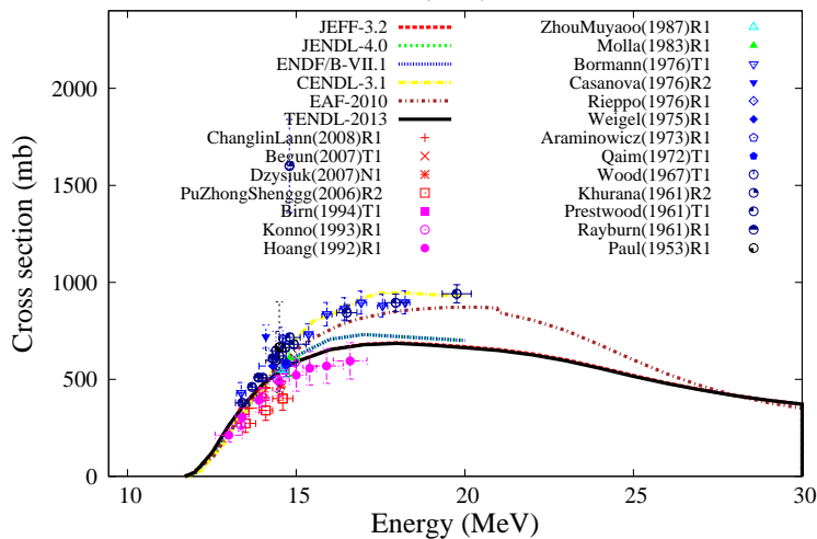
^{76}\text{Ge}(n,2n)^{75}\text{Ge}
