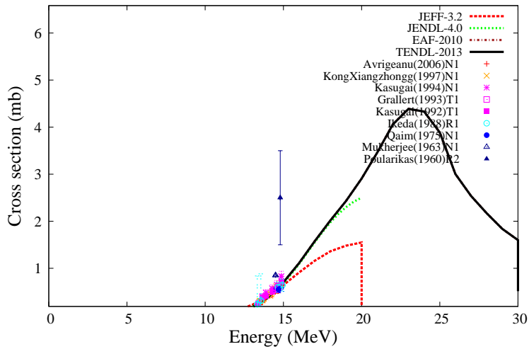
^{187}\text{Re}(n,a)^{184}\text{Ta}
