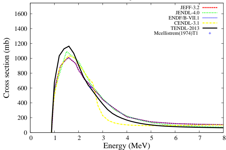
^{98}\text{Mo}(n,n_1)^{98}\text{Mo}
