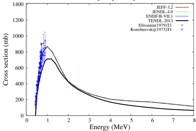
^{202}\text{Hg}(n,n_1)^{202}\text{Hg}
