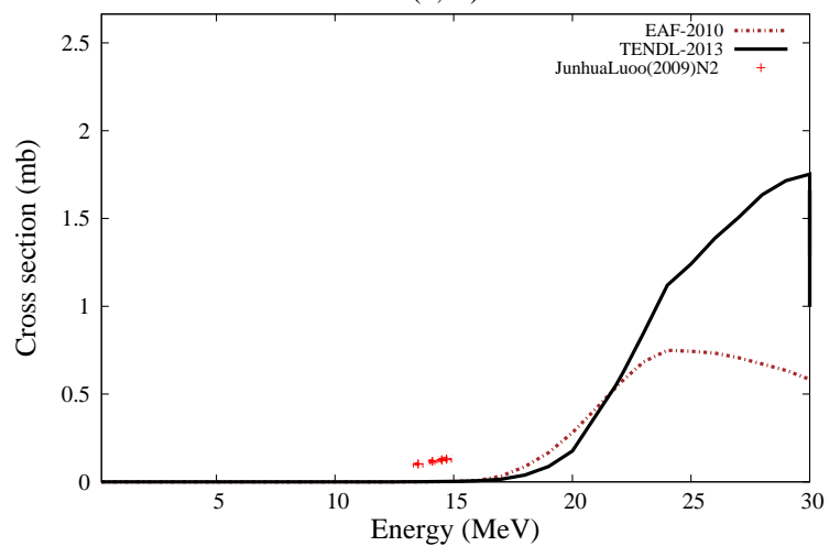
^{181}\text{Ta}(n,n\alpha)^{177\text{m}}\text{Lu}
