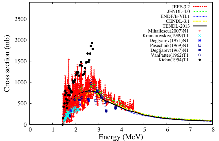
^{55}\text{Mn}(n,n_1)^{55}\text{Mn}
