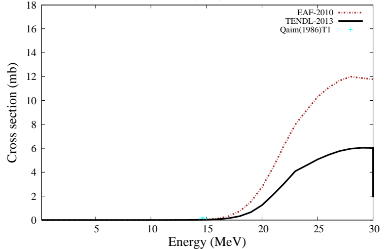
^{181}\text{Ta}(n,n\alpha)^{177\text{m}}\text{Lu}
