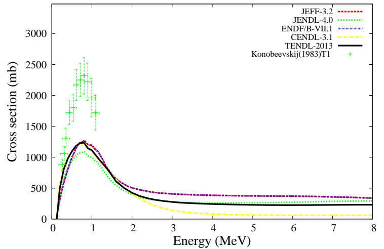
^{162}\text{Dy}(n,n_1)^{162}\text{Dy}
