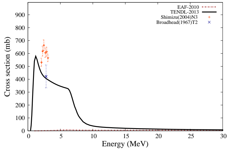
^{181}\text{Ta}(n,n)^{181}\text{Ta}
