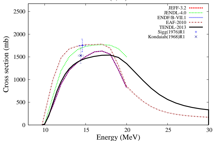
^{128}\text{Xe}(n,2n)^{127}\text{Xe}
