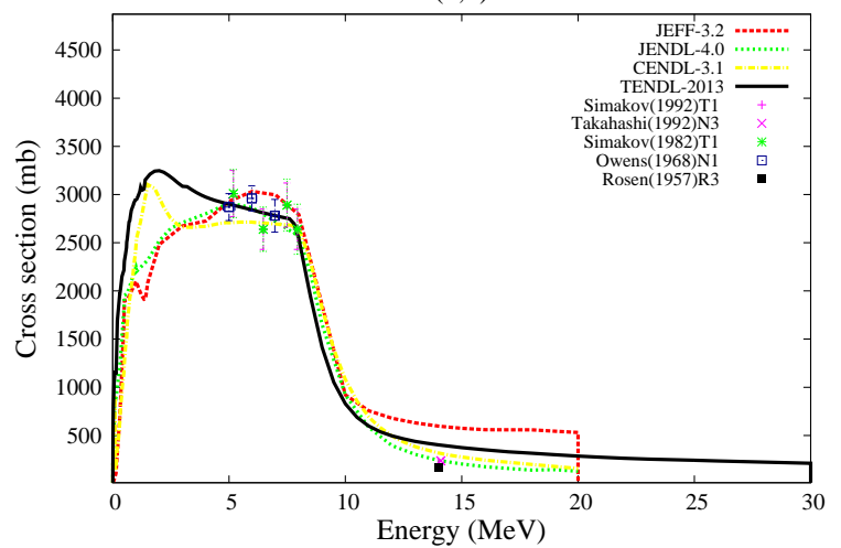
^{183}\text{W}(n,n)^{183\text{m}}\text{W}
