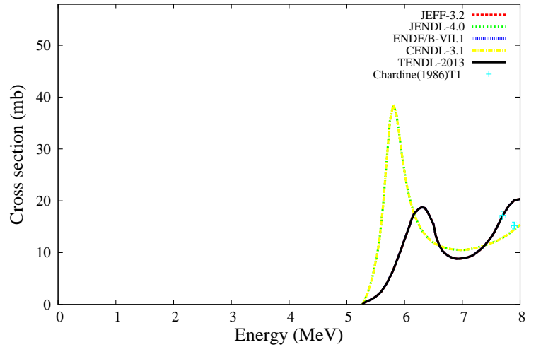
^{23}\text{Na}(n,n_3')^{23}\text{Na}
