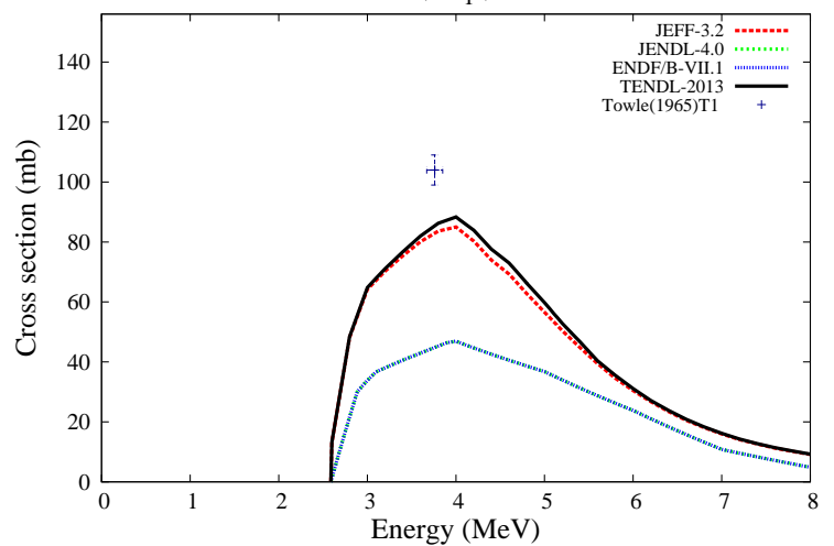
^{39}\text{K}(n,n_1')^{39}\text{K}
