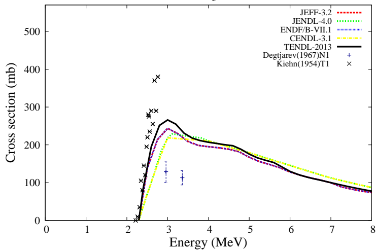
^{27}\text{Al}(n,n_3')^{27}\text{Al}
