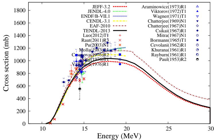
^{70}\text{Ge}(n,2n)^{69}\text{Ge}
