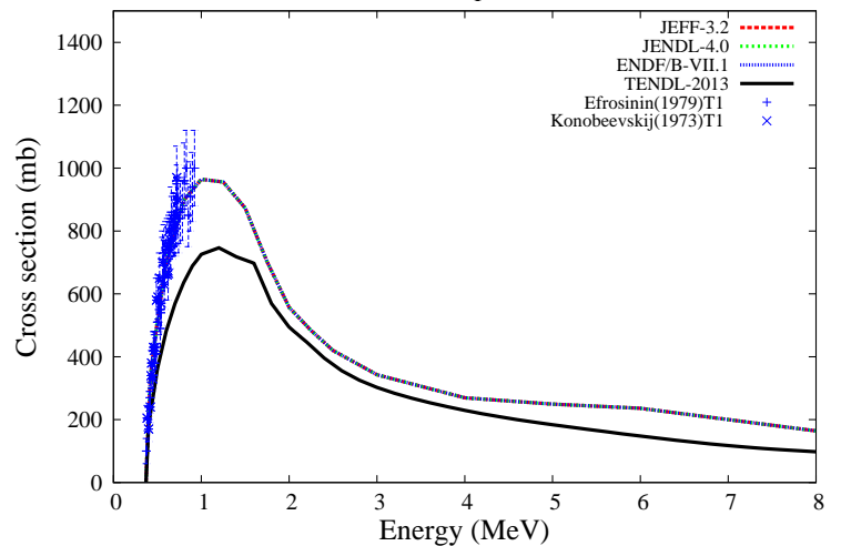
^{204}\text{Hg}(n,n_1)^{204}\text{Hg}
