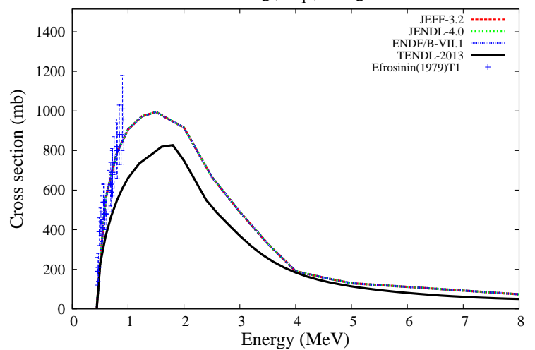
^{204}\text{Hg}(n,n_1)^{204}\text{Hg}
