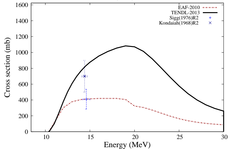
^{128}\text{Xe}(n,2n)^{127g}\text{Xe}
