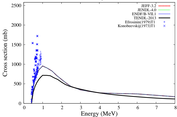
^{202}\text{Hg}(n,n_1)^{202}\text{Hg}
