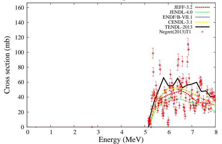
^{28}\text{Si}(n,n_3')^{28}\text{Si}
