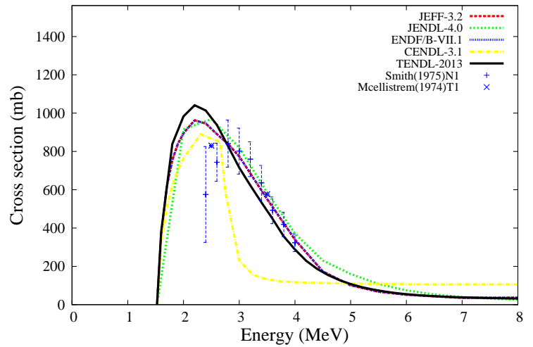
^{96}\text{Mo}(n,n_1)^{96}\text{Mo}
