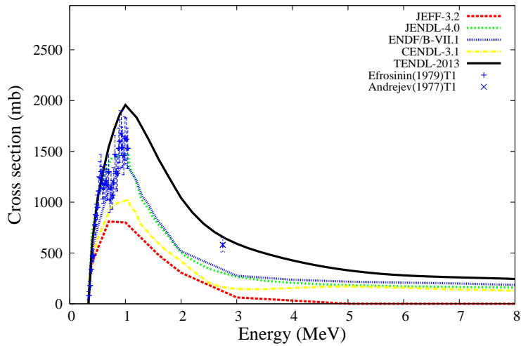
^{154}\text{Sm}(n,n_1)^{154}\text{Sm}
