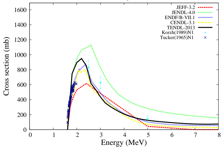
^{140}\text{Ce}(n,n_1)^{140}\text{Ce}
