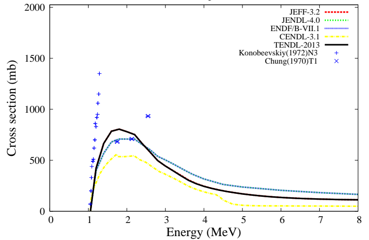
^{74}\text{Ge}(n,n_1')^{74}\text{Ge}
