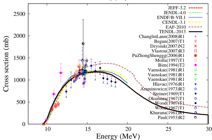
^{76}\text{Ge}(n,2n)^{75}\text{Ge}
