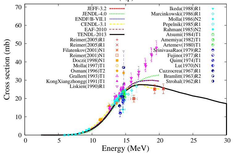
^{96}\text{Mo}(n,p)^{96}\text{Nb}
