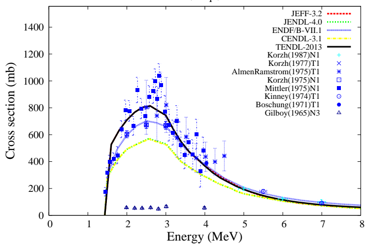
^{54}\text{Fe}(n,n_1)^{54}\text{Fe}
