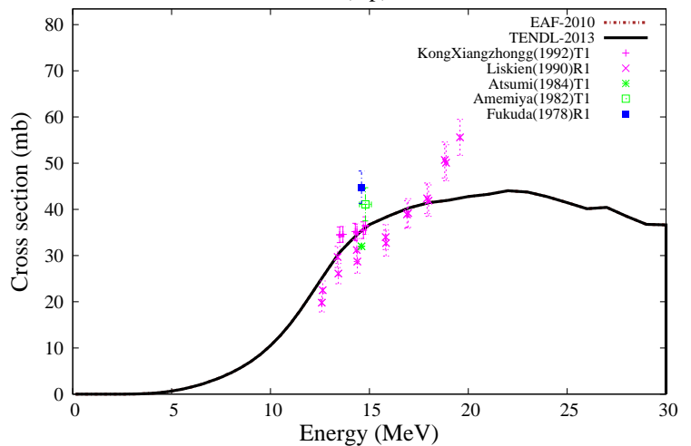
^{96}\text{Mo}(n,p)^{96}\text{Nb}
