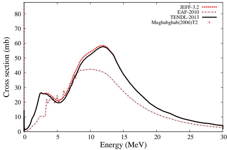
^{39}\text{K}(n,a)^{36}\text{Cl}
