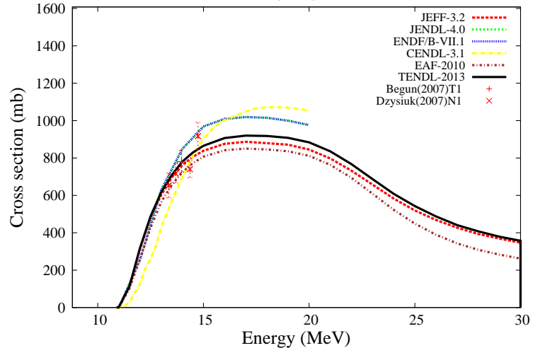
^{76}\text{Ge}(n,2n)^{75g}\text{Ge}
