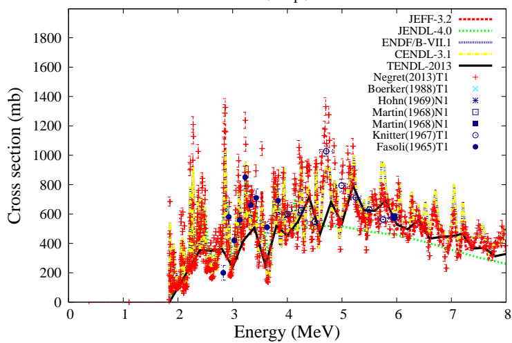
^{32}\text{S}(n,n_1')^{32}\text{S}
