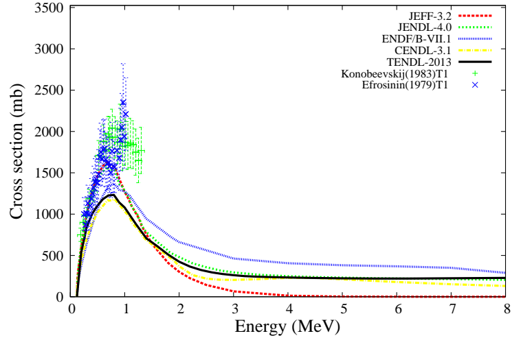
^{154}\text{Gd}(n,n_1)^{154}\text{Gd}
