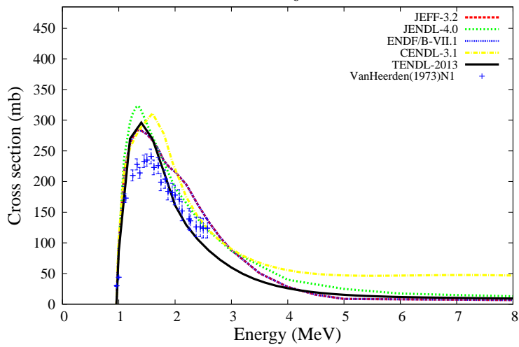
^{191}\text{Ir}(n,n_6')^{191}\text{Ir}
