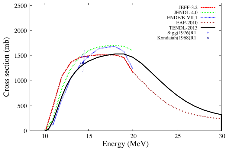
^{128}\text{Xe}(n,2n)^{127}\text{Xe}
