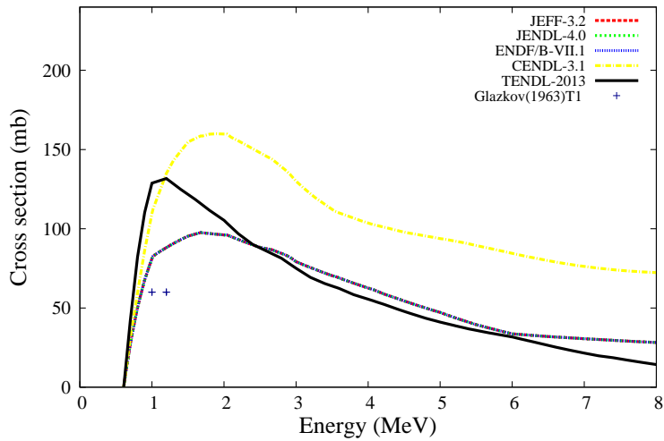
^{28}\text{Si}(n,n_1')^{28}\text{Si}
