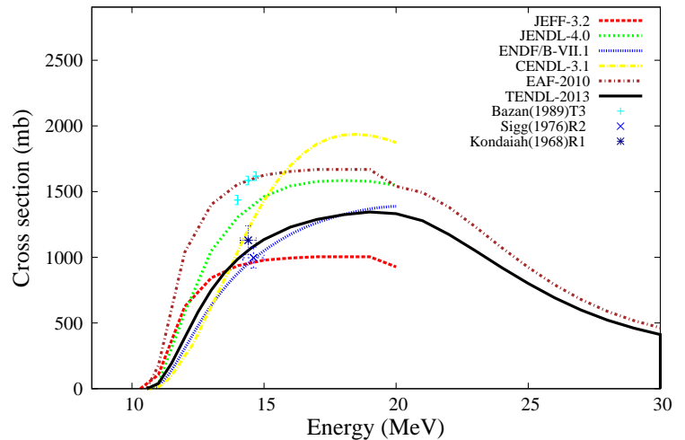
^{126}\text{Xe}(n,2n)^{125m}\text{Xe}
