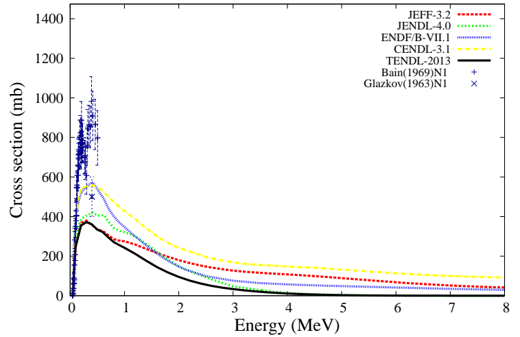
^{138}\text{Ba}(n,n_1)^{138}\text{Ba}
